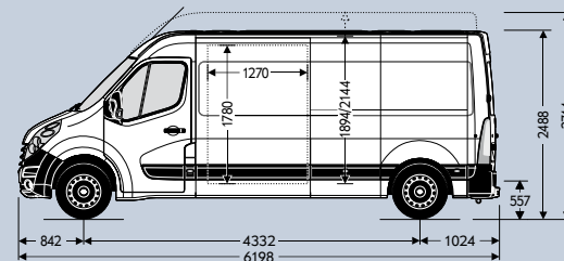
L3H2/H3 FWD
